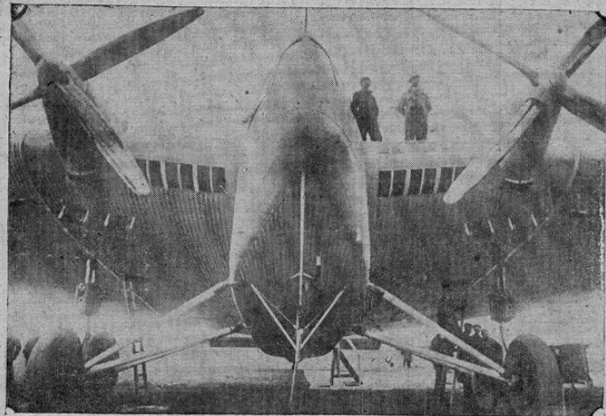
Esta foto, tomada en Dessau, Alemania, muestra el avión Junkers G-38, el más grande aeroplano construido. Tiene cuatro motores. Las personas que se ven sirven para mostrar el tamaño del aparato
