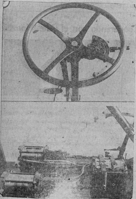
J. H. Newmark, de Nueva York, ha perfeccionado un aparato que permite, oprimiendo simplemente un botón, cambiar las marchas de un carro
