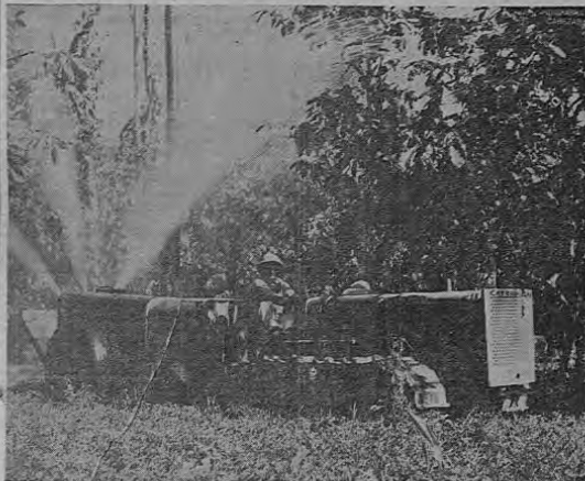
En el grabado aparece una de nuestras excepcionales unidades de FUMIGACION A ALTA PRESION, compuesta de una eficiente y moderna bomba JOHN DEERE de 700 libras de presión remolcada por un inigualable y potente tractor D-2 CATERPILLAR en la Hacienda Theorama de Río Hondo, Limón.
