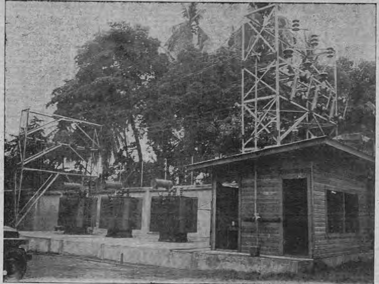
Nueva Sub-estación de Puntarenas Capacidad: 3.000 K. W.
