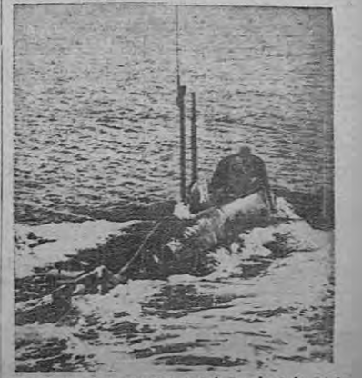
El "X-1", primer submarino diminuto de la Escudera de los Estados Unidos puesto a prueba últimamente. El submarino de 30 pies de longitud, que desplaza 15 toneladas, fue construido para ayudar a probar las defensas de nuestros puertos costeros y está adscrito a la Base Naval de Submarinos de Estados Unidos en New London, Connecticut. La nave opera bajo el mando del Teniente Kevin Hamilton, de Adelphi, Maryland, y lleva solamente cuatro tripulantes. — Teléfono de la (7).
