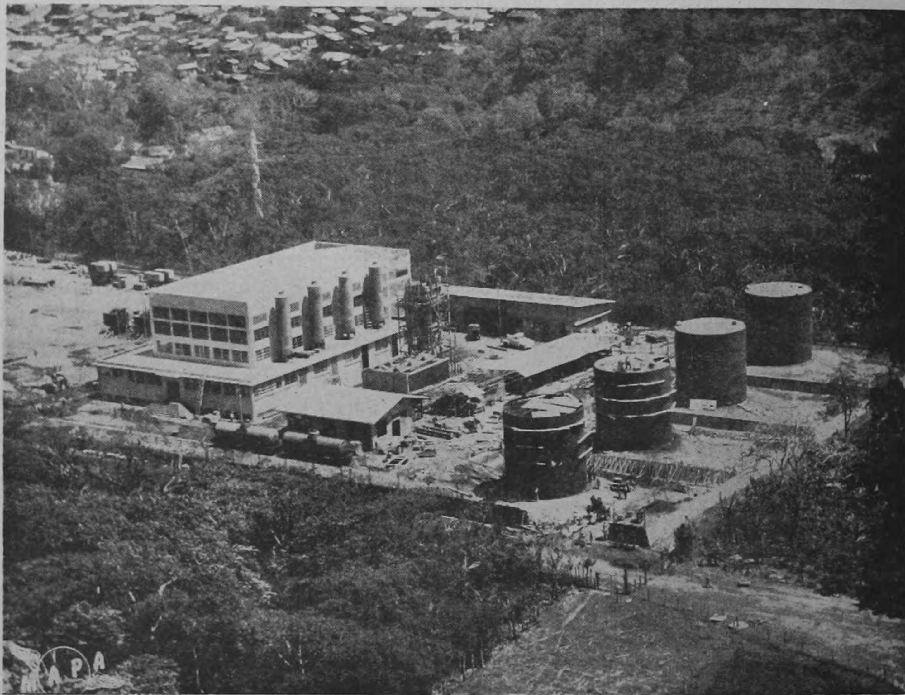
Vista aérea del conjunto que constituye la Central Diesel Eléctrica de Colima. A la izquierda se ve el edificio de casa de máquinas con sus grandes chimeneas, otras obras al centro, y a la derecha los tanques para combustible, con capacidad para 150 mil galones cada uno.
