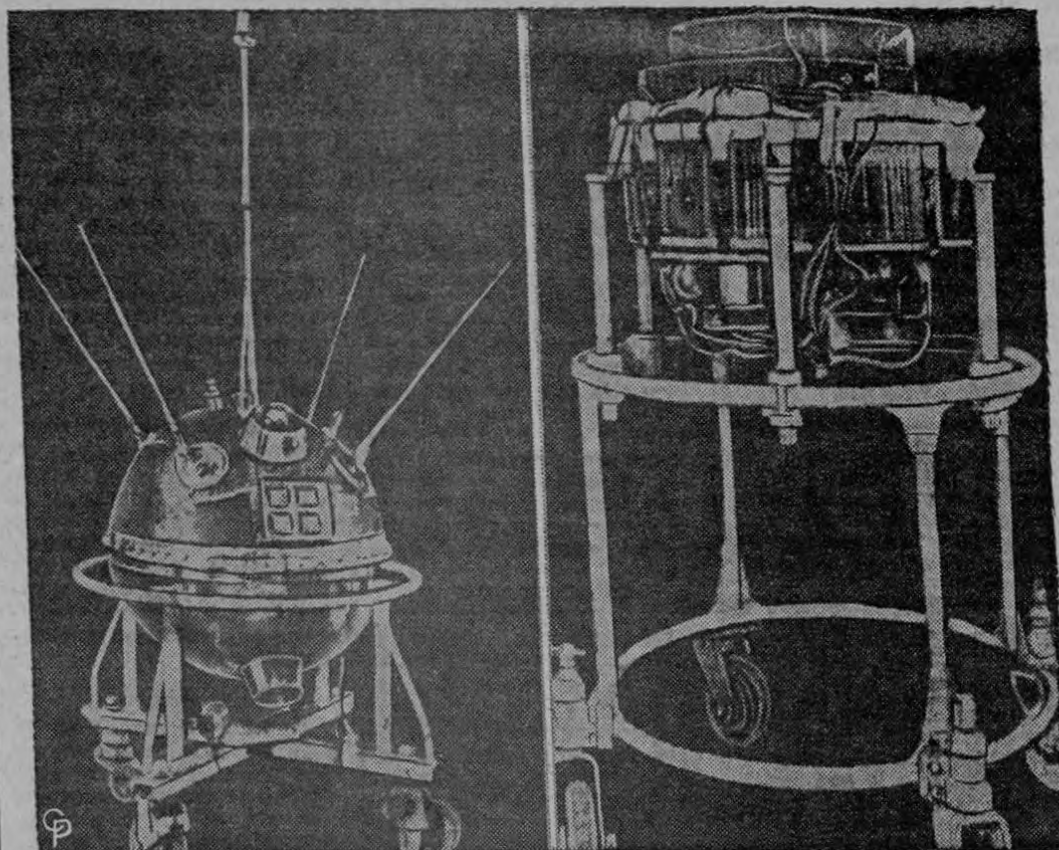
Fotografías del periódico comunista Pravda muestran a la cápsula de instrumentos (izquierda) del cohete cósmico soviético. Los rusos dicen que un sistema de orientación automático puso al proyectil en órbita alrededor del sol. A la derecha la batería y unidad eléctrica del cohete, que fue lanzado verticalmente desde un lugar de la Unión Soviética que no ha sido revelado.
