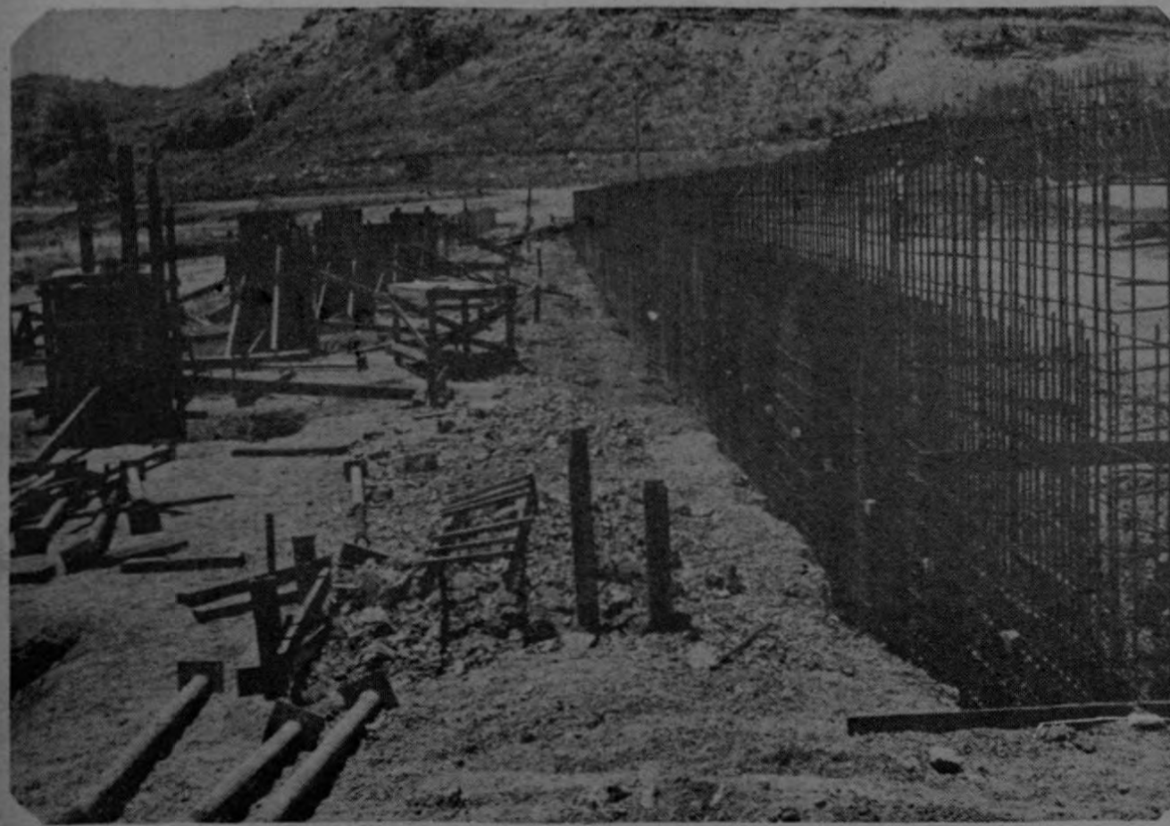
Los cimientos de la nave que almacenará el clinker se han chorreado en buena parte y la estructura de hierro se empieza a levantar, como se puede observar en la gráfica.
