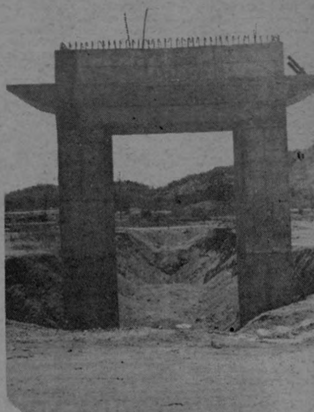
Una de las columnas que soportarán el horno de 60 metros de longitud y 4.26 metros de diámetro.
