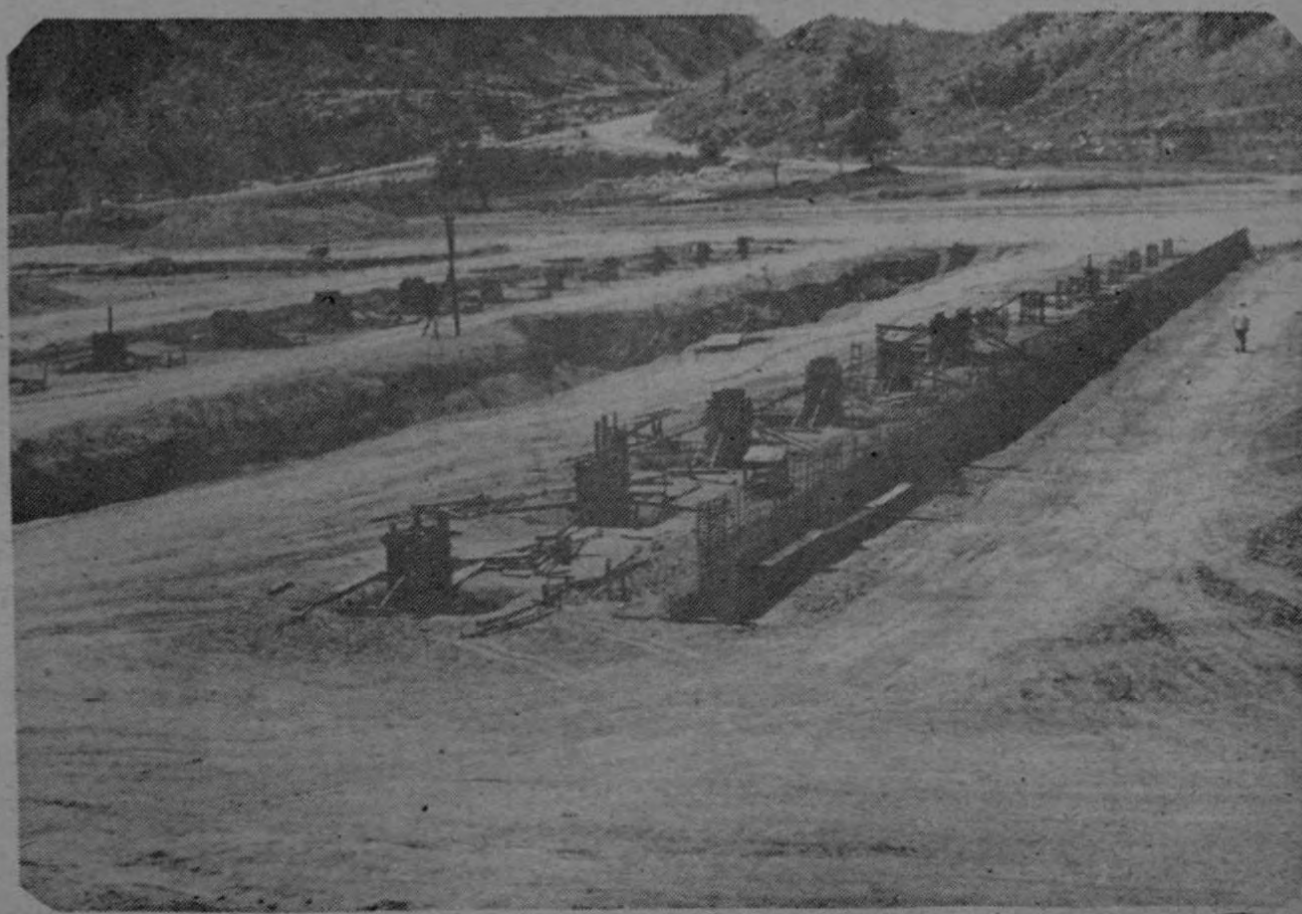
Por otra parte, la nave de materias primas, una vez compactado el piso, también se empieza a levantar, con la construcción de los cimientos para las columnas que soportarán paredes y techo.
