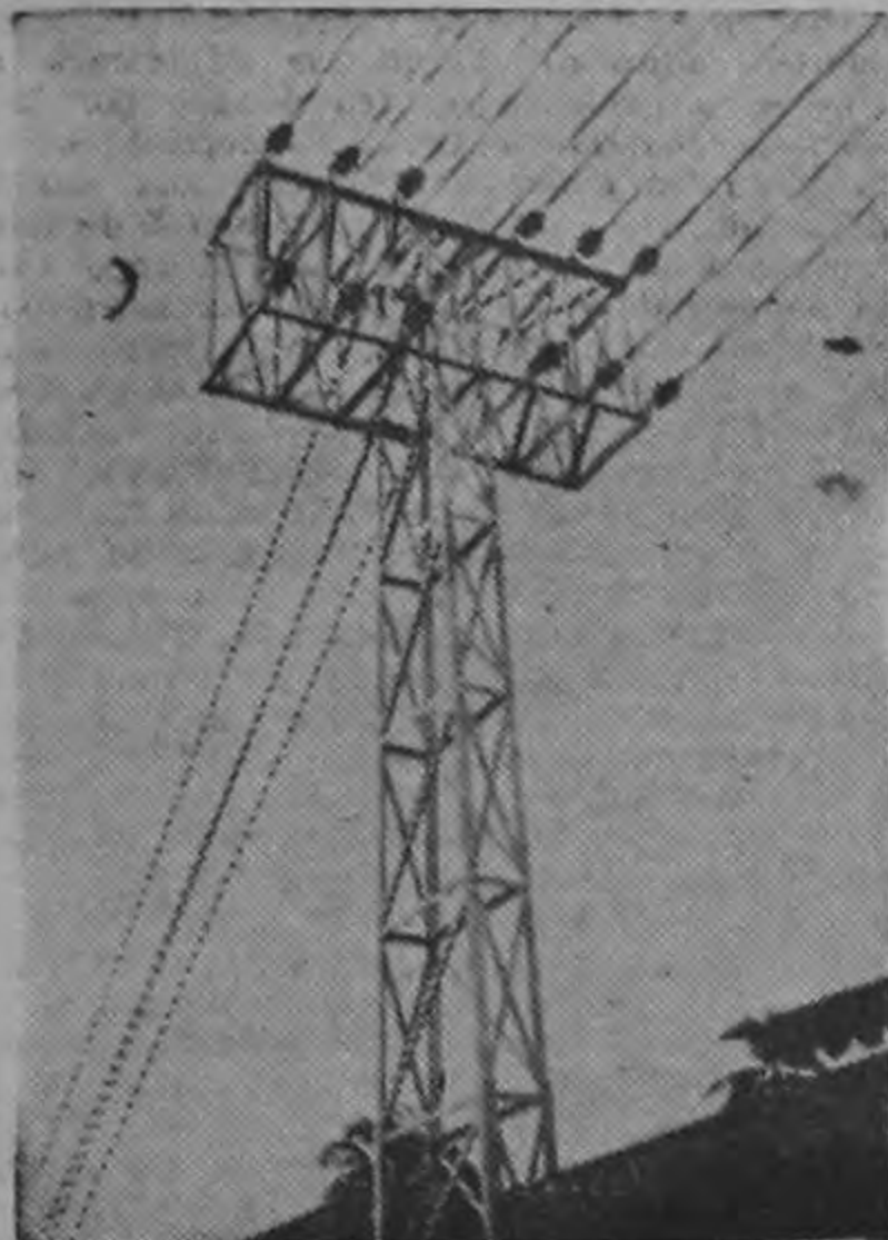
Torre de remate con cuatro circuitos primarios de distribución. La Torre que se indica con cuatro circuitos de distribución ha mejorado en forma notable los servicios eléctricos.
